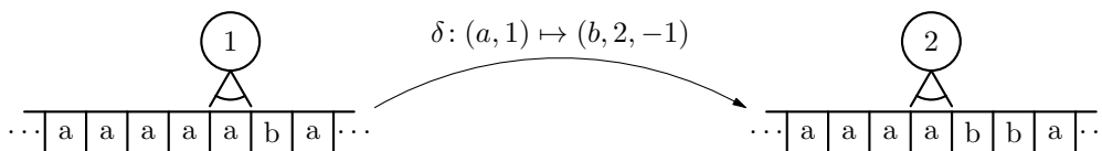
Рис. 1: Такт работы машины Тьюринга
