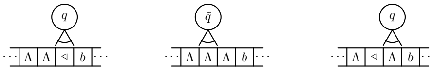
Рис. 4: Сдвиг левого ограничителя рабочей зоны
