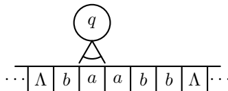
Рис. 2: Конфигурация МТ: слово bqaabb
